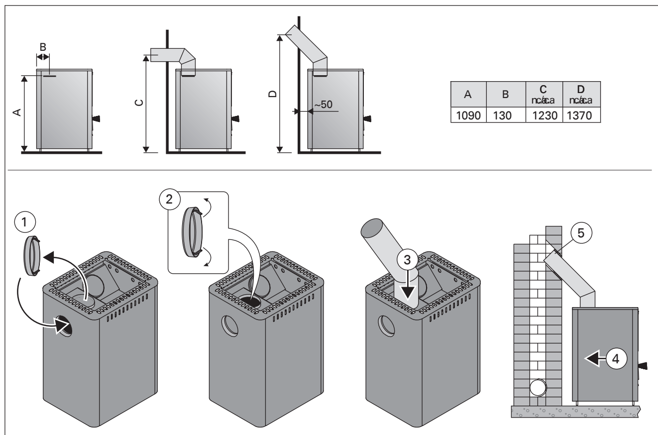
Obrázek 9. Připojení kamen ke zděři ve zdi z horního otvoru (všechny rozměry jsou uvedené v milimetrech) Rysunek 9. Podłączenie pieca do komina górnym otworem (wymiały w milimetrach)
