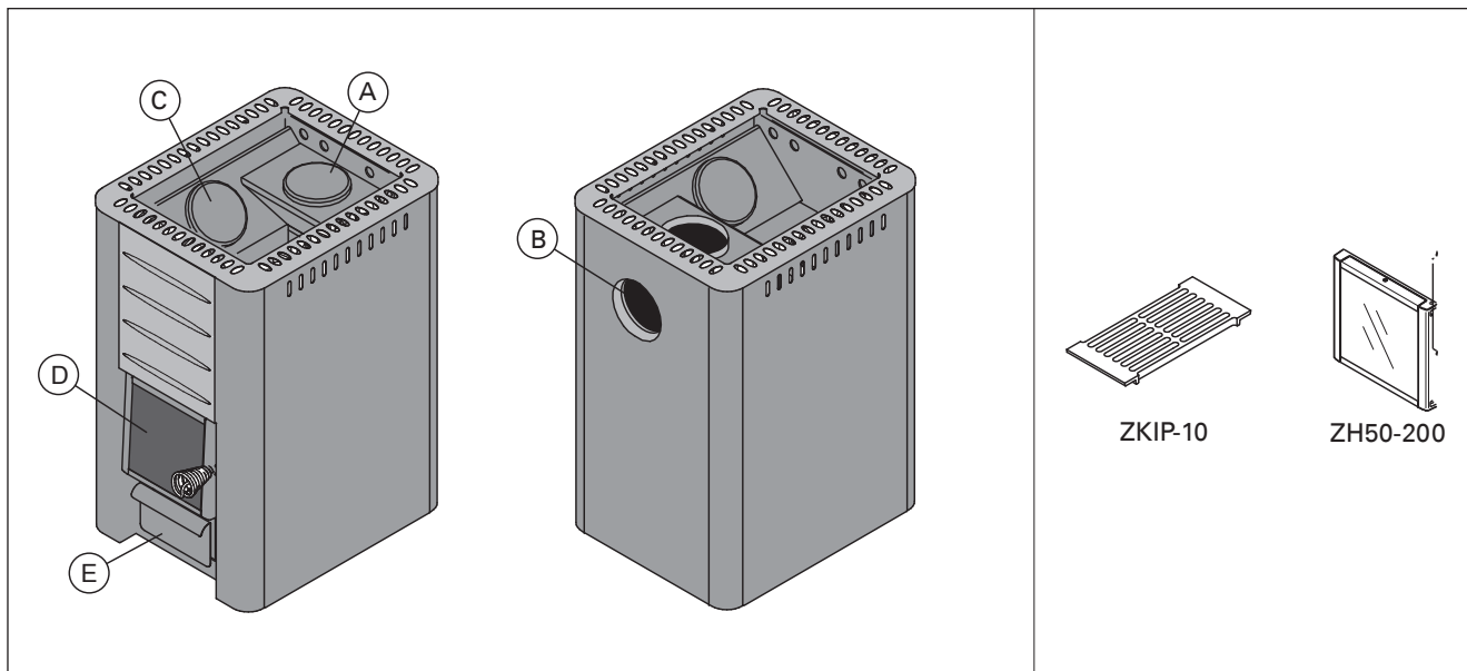
Kuva 1. Kiukaan osat
