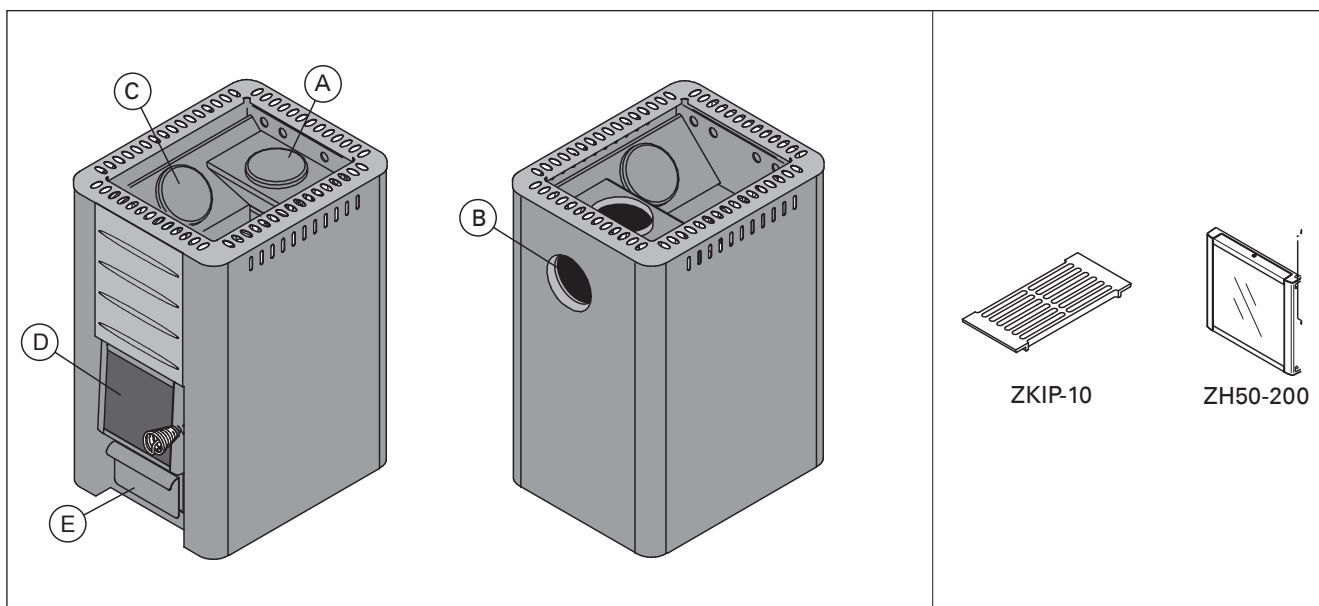
Obrázek 1. Součásti kamen Rysunek 1. Części pieca
