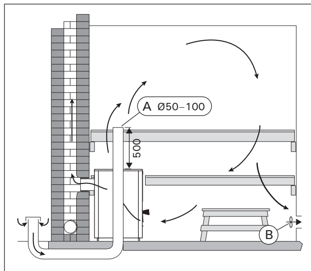
Kuva 4. Koneellinen ilmanvaihto Bild 4. Maskinell ventilation
