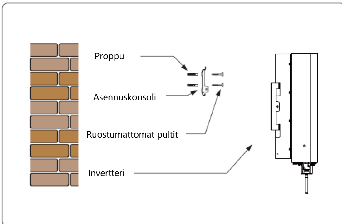
Kuva 4.2.1 Havainnekuva invertterin seinään asennuksesta.
