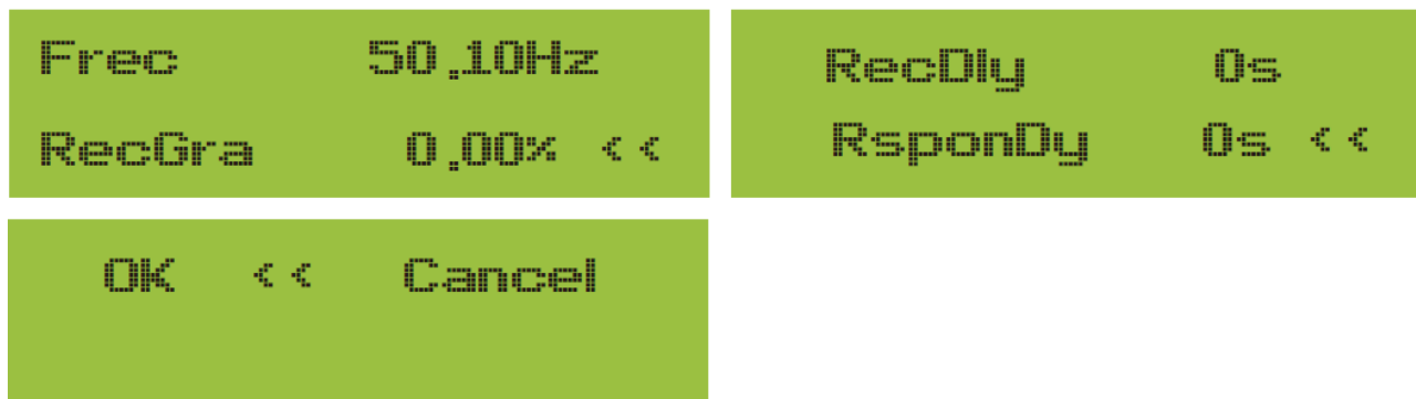
Kuva 8.4.11 OF-Derate" tarkoittaa suomeksi " ylitaajuuden tehon rajoitus ". Tämä viittaa siihen, kuinka paljon invertterin tehoa vähennetään ylitaajuusolosuhteissa.
