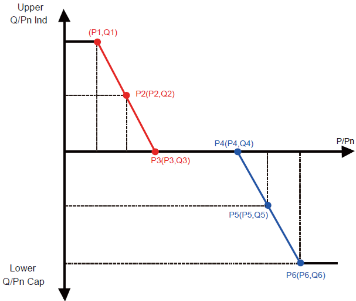
Kuva 8.4.17 Invertterin loistehon tuotantoa ohjataan invertterin pätöteholla. Loistehon säätökäyrä Q(P) -tilassa.
