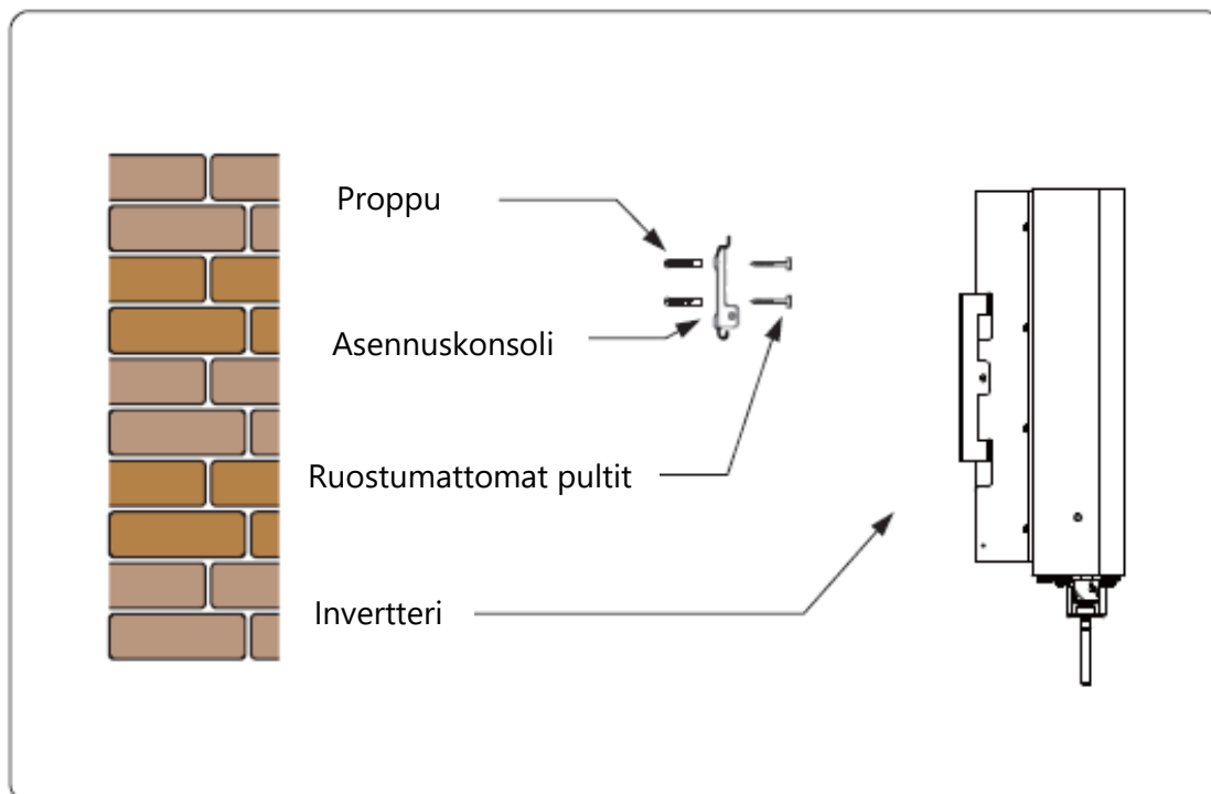
Kuva 4.2.1 Havainnekuva invertterin seinään asennuksesta.
