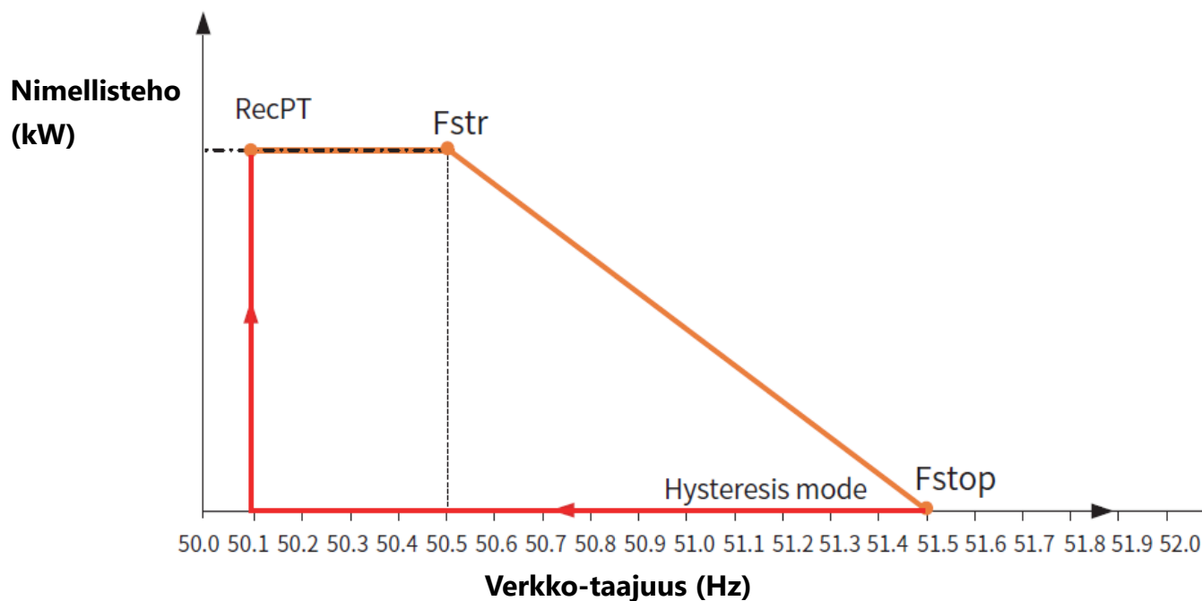
Kuva 8.4.8 Frq-Watt-tila ylitaajuusolosuhteissa.
