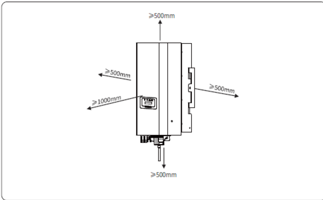
Kuva 4.1.3 Invertterin asennuksen vaatima tilantarve eri suuntiin.
