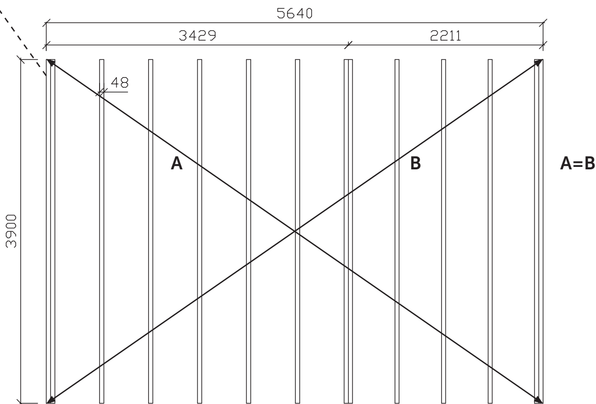
Perustuspuiden asettelu - Monteringen av grundbalkarna Montering av grunnbjelkene - Monteringen af fundamentbjælkerne Assembling of foundation beams - La pose des solives
