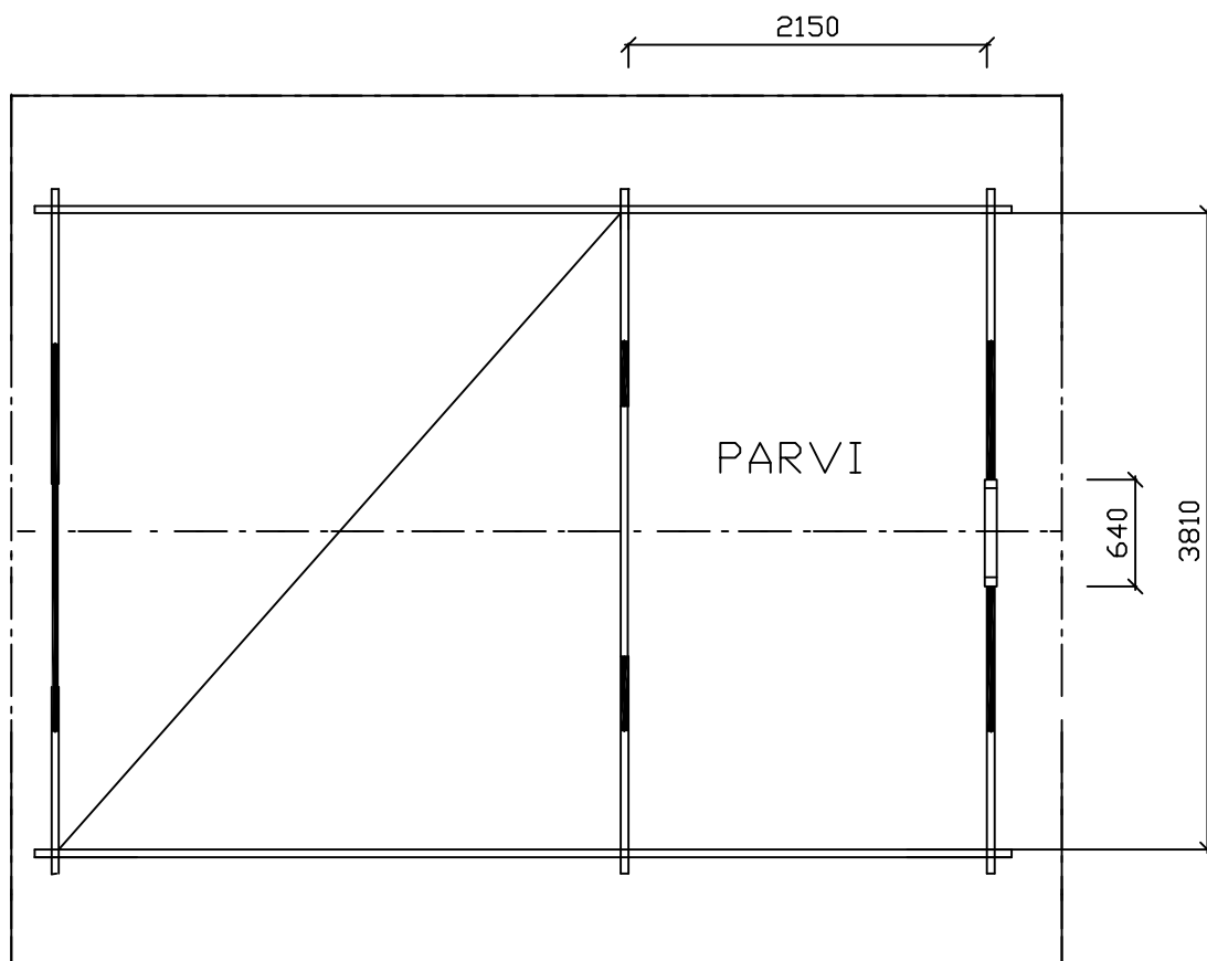
PÖHJAPIIRUSTUS PARVI
