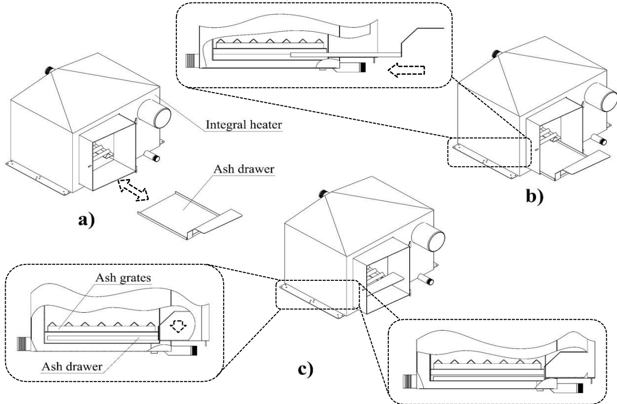
Kuva 7. Tuhkaritilän sijoittaminen (Kokoamisvaihe 5).
