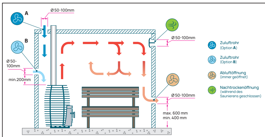
Abbildung 12. Mechanische Belüftung einer Holzbeheizten Sauna.
