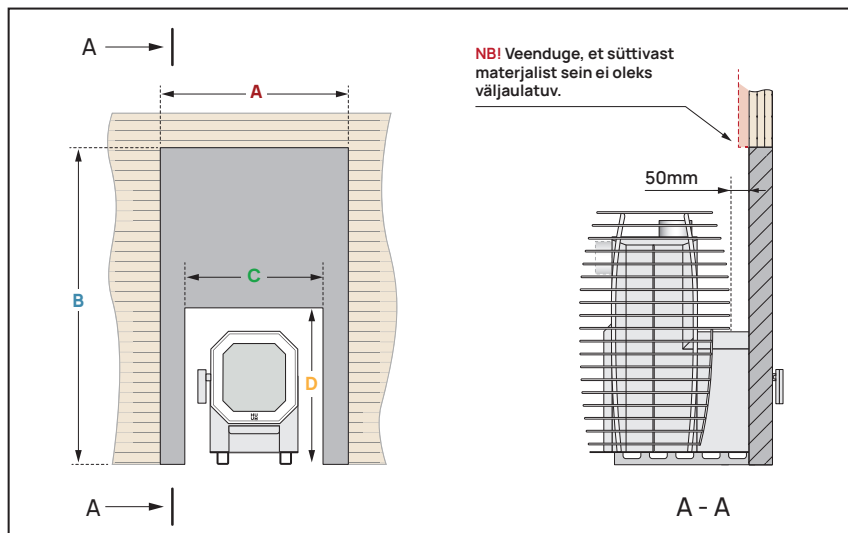
Joonis 9. HIVE Flow LS ja Flow Mini LS saunaahju paigaldamine läbi sein.
