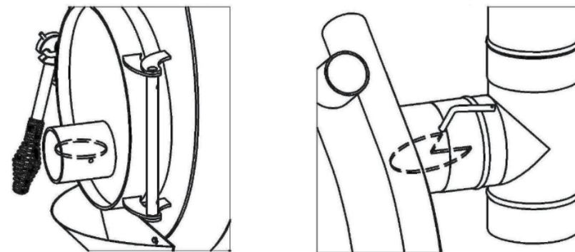
Joonis 11. Siibrite asend süütamisel või küttepuude lisamisel (intensiivne režiim)
