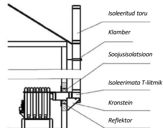
Joonis 6. Lõõri paigaldamine läbi seina
