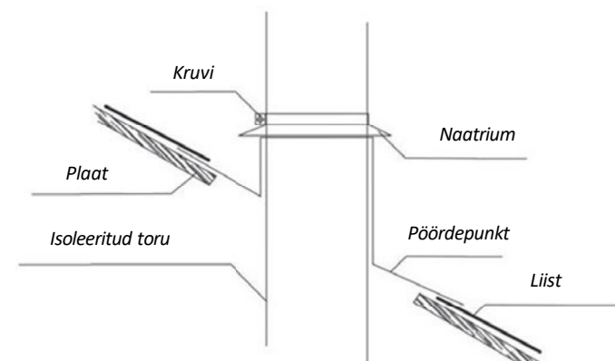
Joonis 9. Lõõri paigaldus läbi katuse
