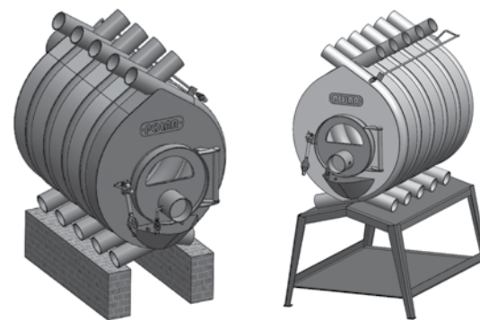
Joonis 2. Ahju paigaldamise võimalused
