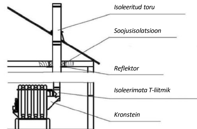
Joonis 5. Lõõri paigaldamine läbi lae
