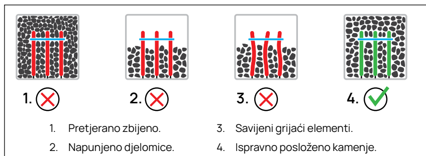
Slika 7 Postavljanje kamenja u DROP 4 i DROP 6, s tri grijaća elementa.
