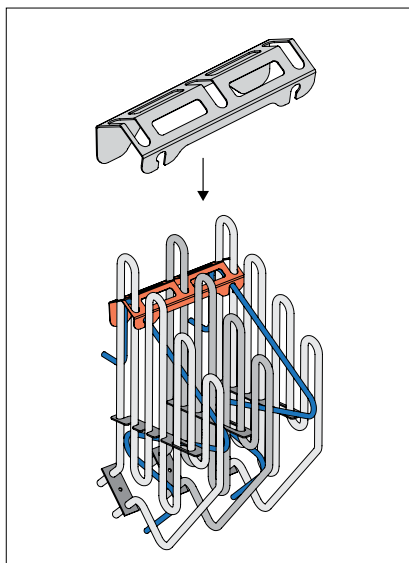
3 pav. HUUM DROP 4 ir 6 su 3 kaitinimo elementais laikiklio montavimas.
