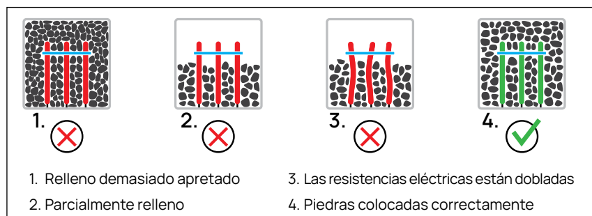
Figura 7. Colocación de las piedras en DROP 4 y DROP 6 con 3 elementos calefactores.
