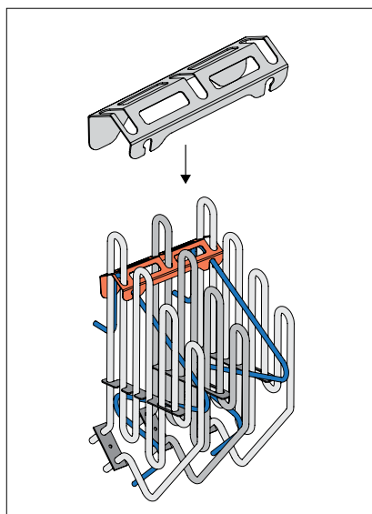
Figura 3. Instalación del retenedor de HUUM DROP 4 y 6 con 3 resistencias eléctricas.
