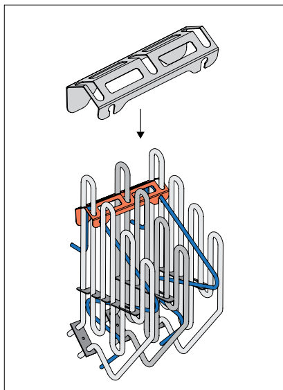
3. attēls HUUM DROP 4 un 6 atdalītājrēžģa uzstādīšana ar 3 sildelementiem.
