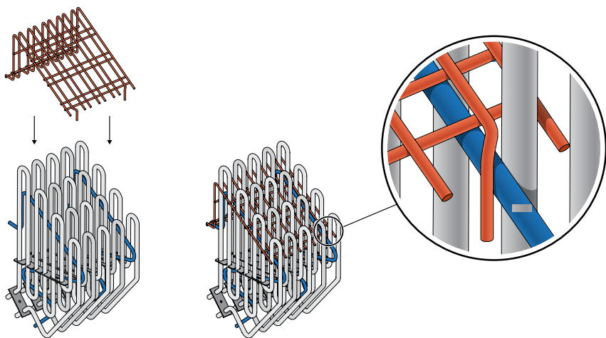
5. attēls HUUM DROP 9 atdalītājrēžģa uzstādīšana ar 5 sildelementiem.
