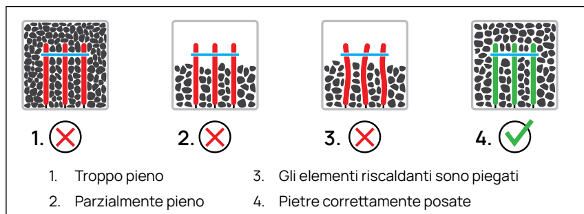
Figura 7. Posizionamento delle pietre in DROP 4 e DROP 6 con 3 elementi riscaldanti.
