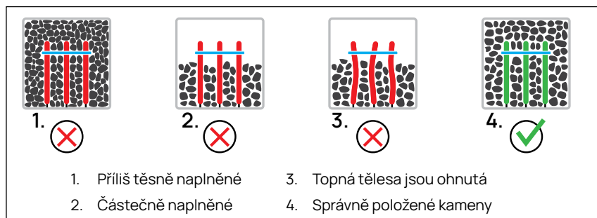
Obrázek 7. Umístění kamenů do modelů DROP 4 a DROP 6 se 3 topnými tělesy.
