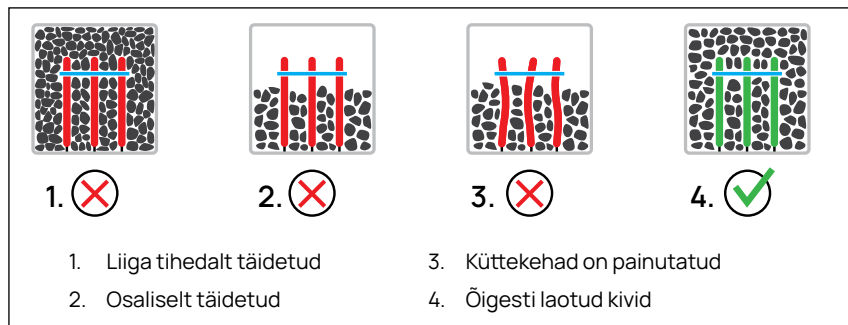
Joonis 7. Kivide ladumine 3 küttekehaga kerisesse DROP 4 ja DROP 6.
