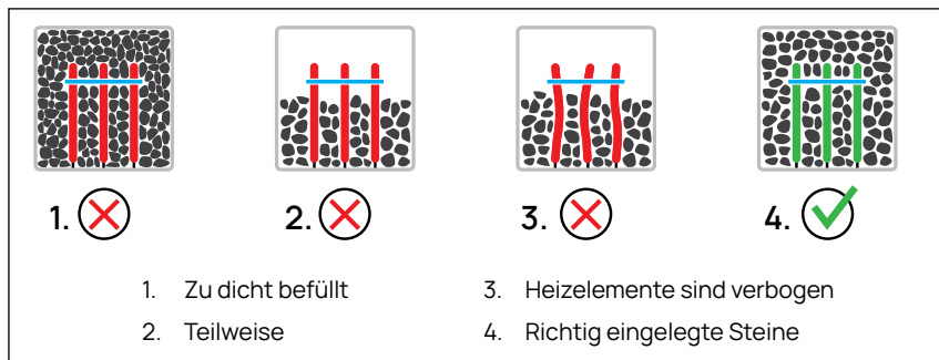
Abbildung 7. Platzieren der Steine in DROP 4 und DROP 6 mit 3 Heizelementen.
