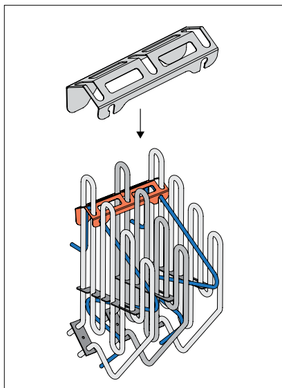
Slika 3 Instaliranje nosača za HUUM DROP 4 i 6, s tri grijaća elementa.
