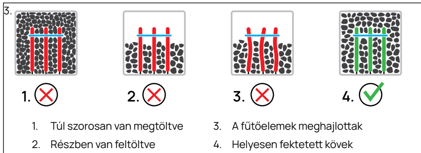
7. ábra: A kövek elhelyezése a DROP 4 és a DROP 6 fűtőberendezésben 3 fűtőelem esetében.
