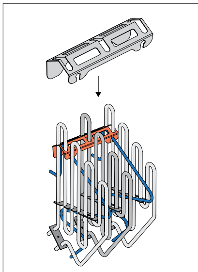
Obrázek 3. Instalace držáku HUUM DROP 4 a 6 se 3 topnými tělesy.
