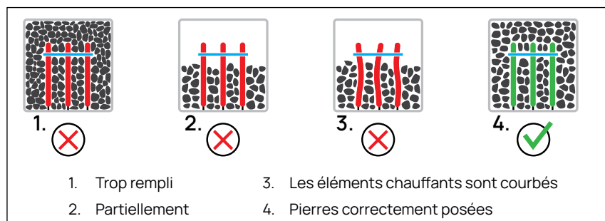
Figure 7. Placer les pierres dans DROP 4 et DROP 6 avec 3 éléments chauffants.
