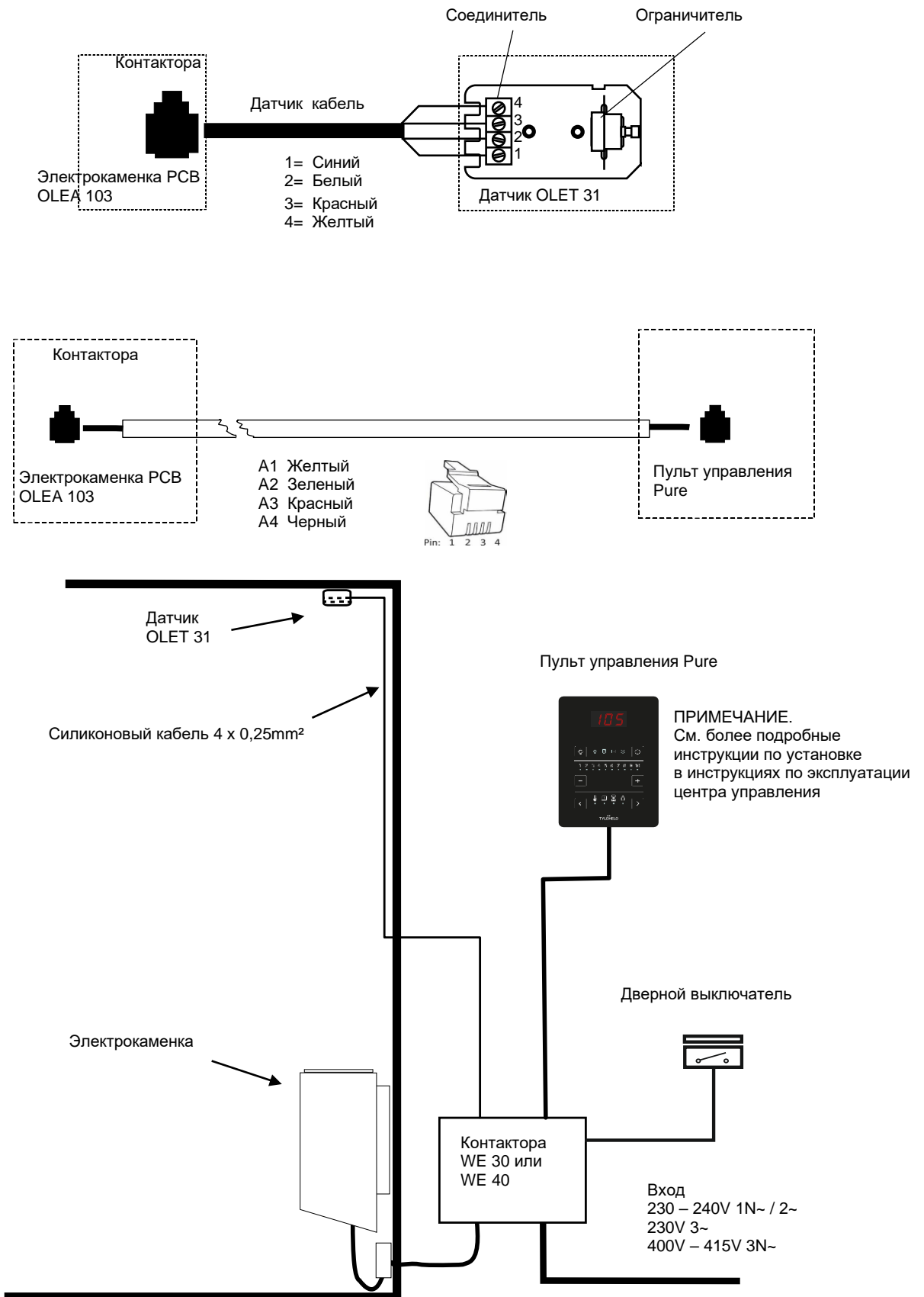
Рисунок 11 Принципиальная схема с пультом Pure
