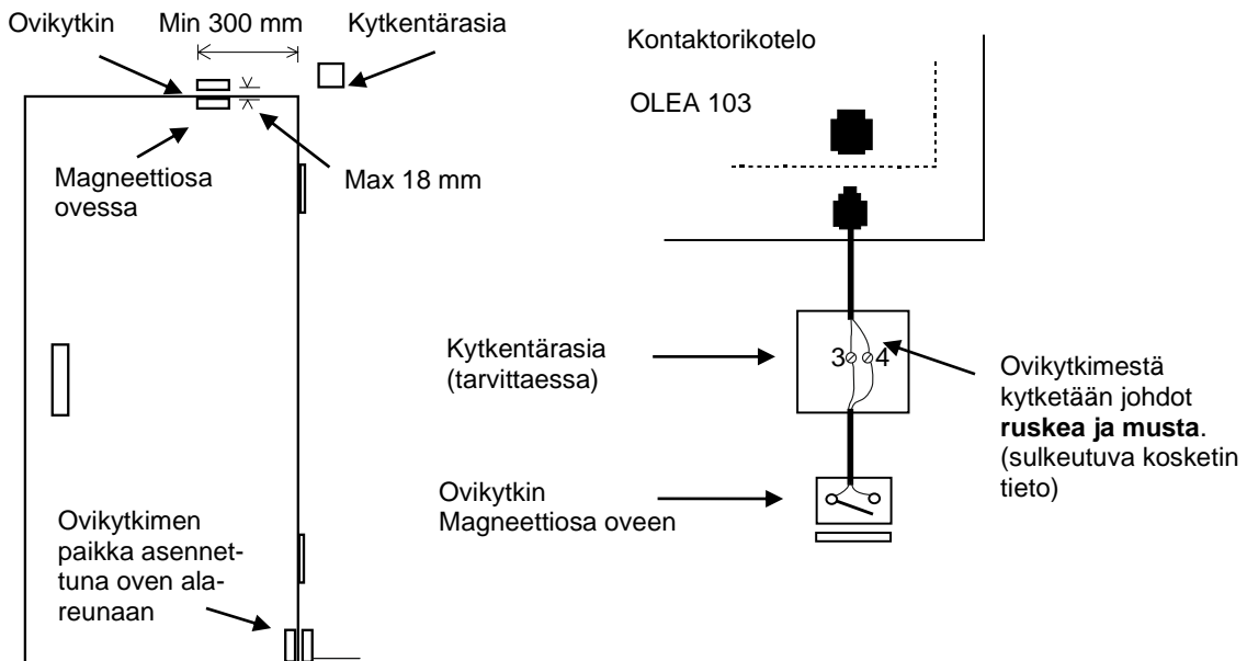
Kuva 7. Ovikytkimen asennus
