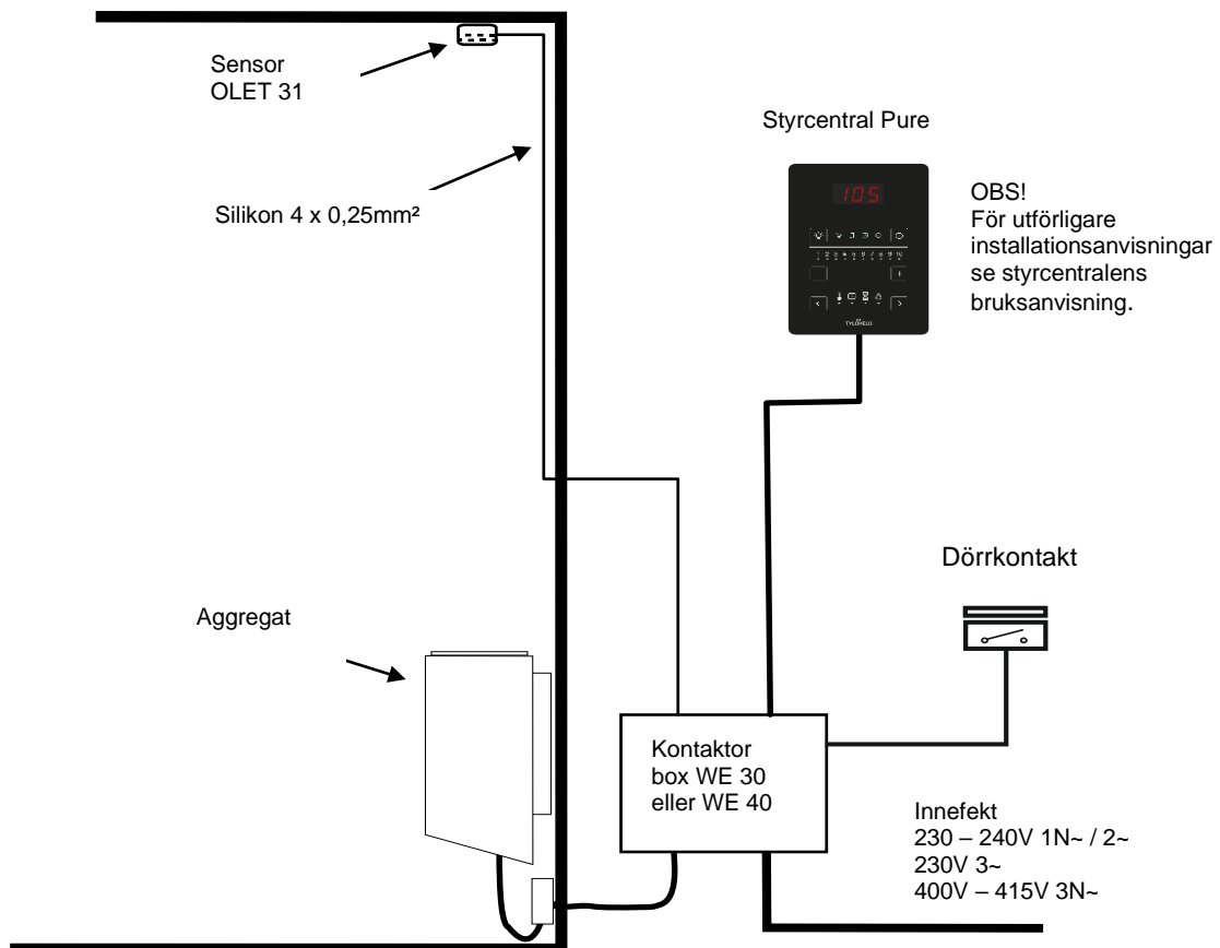
Bild 11 Principskiss
