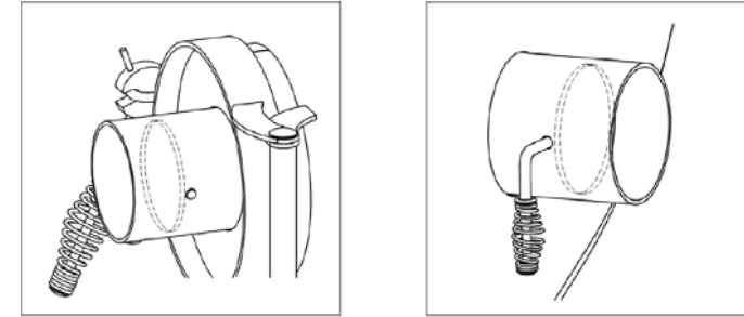
Kuva 7. Peltien asennot ensisijaisessa lämmitystavassa (taloudellinen lämmitys)
