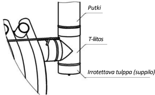
Kuva 3. Asennus T-liitos tulpalla (suppilo)
