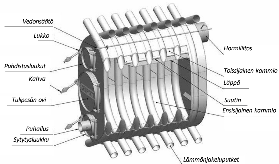
Kuva 1. Lämmitysuuni
