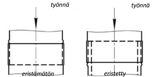
Kuva 2. Hormiputkien liittäminen toisiinsa
