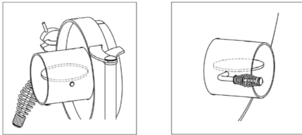
Kuva 6. Peltien asento lämmitysuunia sytytettäessä ja puita pesään lisättäessä (intensiivinen lämmitys)
