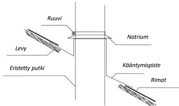
Kuva 4. Hormin asennus katon läpi
